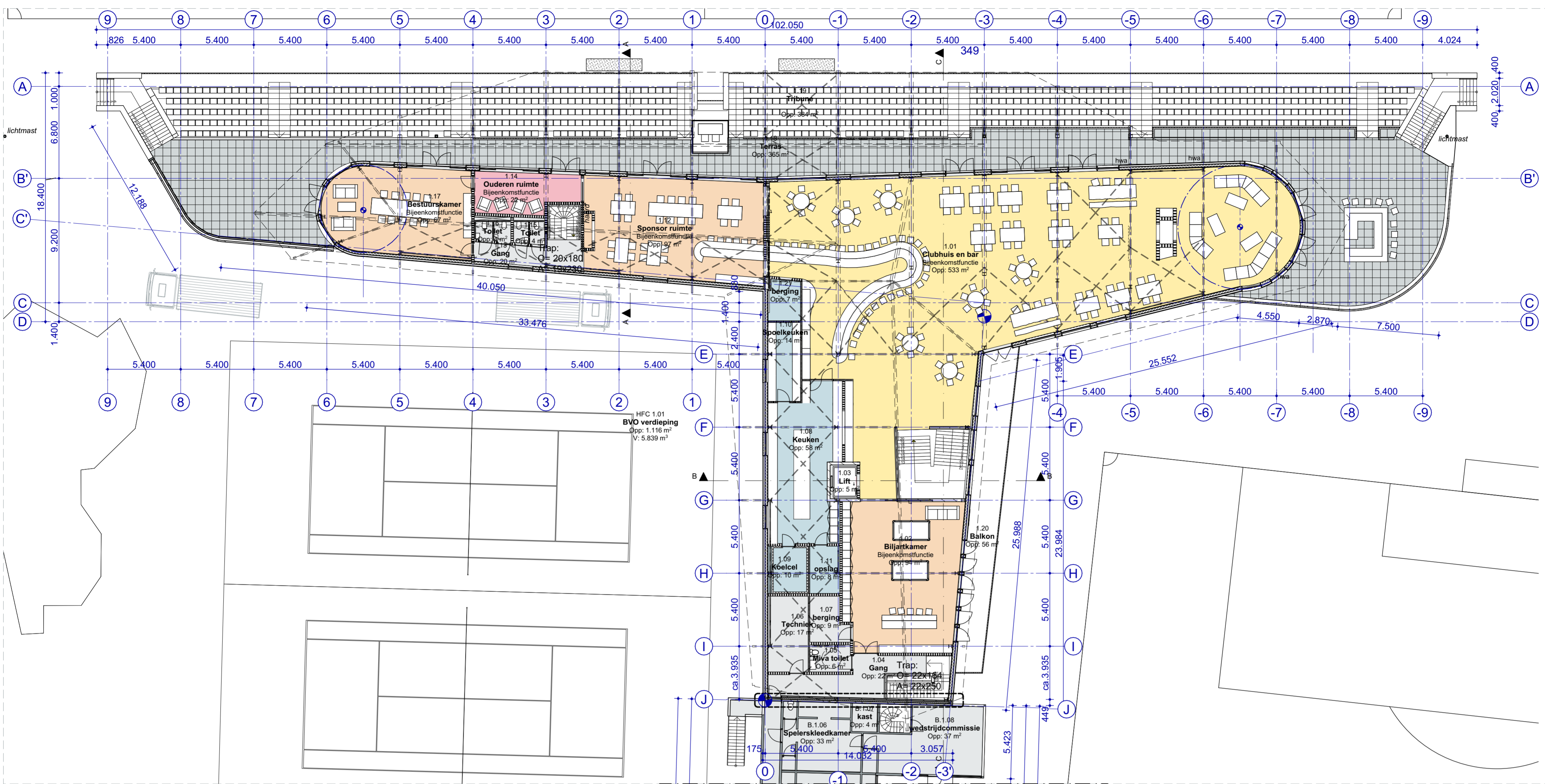
Eerste etage bouwaanvraag versie
